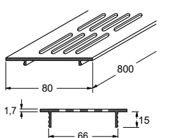
Lüftungsgitter
