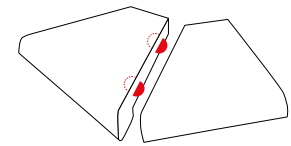
Gehrungsverbindung mit Lamellos**
