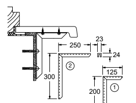
Konsolen
