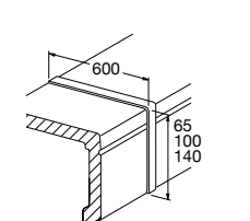
Fensterbank- Verbindungsprofile
